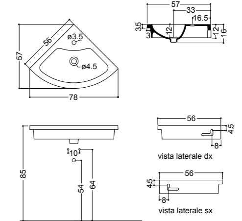
ART. WS323 lavabo angolare incasso, sospeso e appoggio 57 monoforo corner inset, wallhung and overtop basin 57 1/hole
