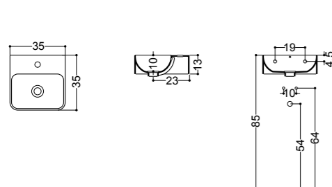
ART. WS103 02C lavabo 35 da appoggio e sospeso monoforo 02C overtop or wall-hung basin 35 1/hole
