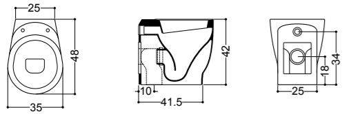
ART. 26014 vaso 48 BTW wc 48
