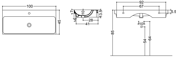
ART. WS109 lavabo sospeso, incasso, da appoggio 100 monoforo wall-hung, inset, overtop basin 100 1/hole
