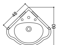
ART. 06035 lavabo angolare 60 monoforo/tre fori su richiesta corner basin 60 1/hole (3/holes upon request)
