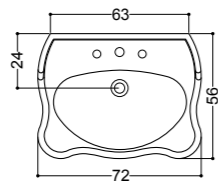
ART. 06030 lavabo 72 a colonna e sospeso monoforo/tre fori su richiesta pedestal/wall-hung basin 72 1/hole (3/holes upon request)
