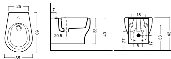
ART. 3625 bidet sospeso 50 monoforo wall hung bidet 50 1/hole
