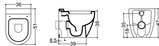
ART. 25014 vaso 51 BTW wc 51
