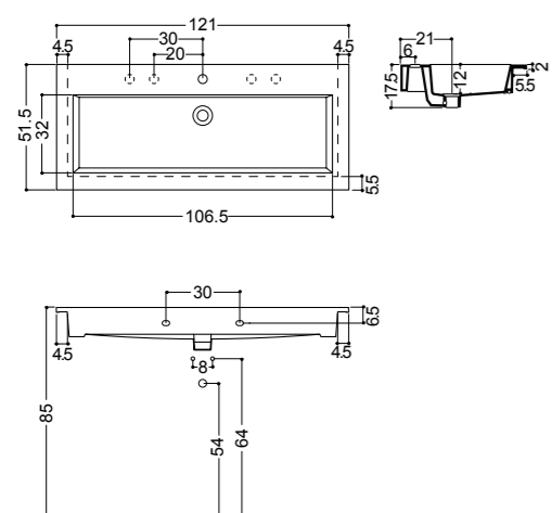
WS331 consolle incasso 121 monoforo inset console 121 1/hole
