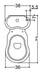
ART. 06012 vaso monoblocco S. floor trap monobloc wc
