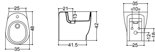
ART. 26022 bidet 48 monoforo BTW bidet 48 1/hole
