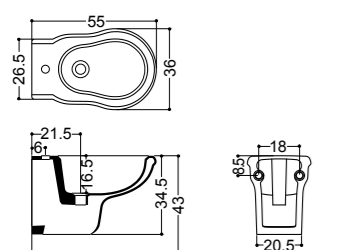
ART. 06070 bidet sospeso monoforo wall-hung bidet 1/hole
