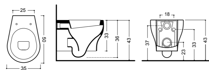
ART. 3615 vaso sospeso 50 wall hung wc 50
