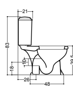
ART. 06013 vaso monoblocco P. wall trap monobloc wc
