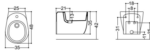
ART. 27022 bidet sospeso 48 monoforo wall-hung bidet 48 1/hole
