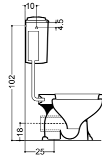
ART. 06010 vaso S. floor trap wc
