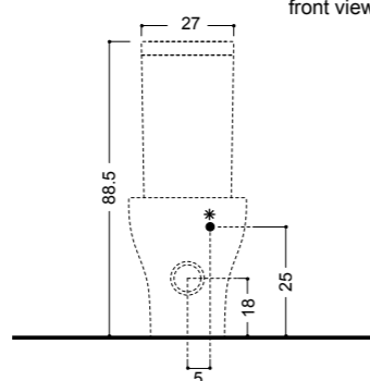
ART. 3681 cassetta monoblocco completa di meccanismo di scarico monobloc cistern chrome dual flush mechanism included
