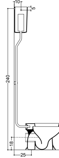
ART. 06010 vaso S. floor trap wc
