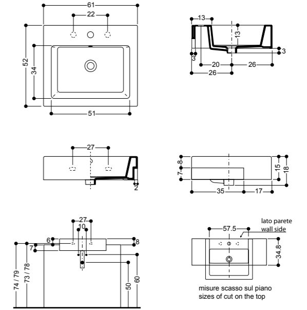
ART. WS044 lavabo semincasso 61 monoforo/tre fori su richiesta semi recessed basin 61 1/hole (3/holes upon request)
