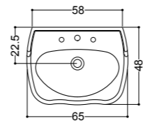
ART. 06031 lavabo 65 a colonna e sospeso monoforo/tre fori su richiesta pedestal/wall-hung basin 65 1/hole (3/holes upon request)
