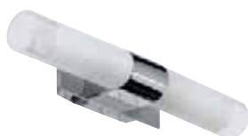
83732 KIO ⊗ 2xG9, 33 W, 230 V, 300x50x75 mm, króm 45.990,-
