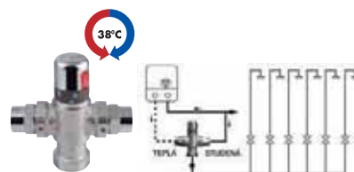
TMTCOM Termosztatikus keverőszelep 4-8 fogyasztóig, 20°-50°C, 1"Fx3/4"F, visszacsapó szeleppel, szűrővel 37.990,-
