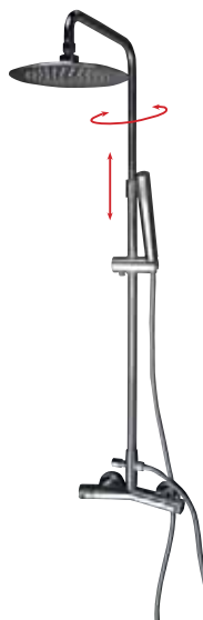
990E Zuhanyoszlop csapterlep nélkül, fej- és kézi zuhannyal, Ø fejuhany: 200 mm állítható magasság: 830-1280 mm 91.990,-
